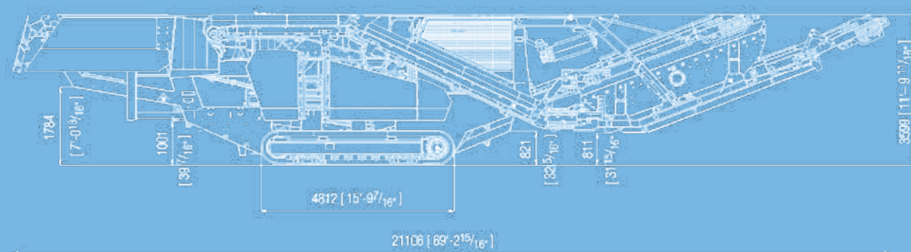
Widok z boku - pozycja transportowa MR 110 Z EVO 2
