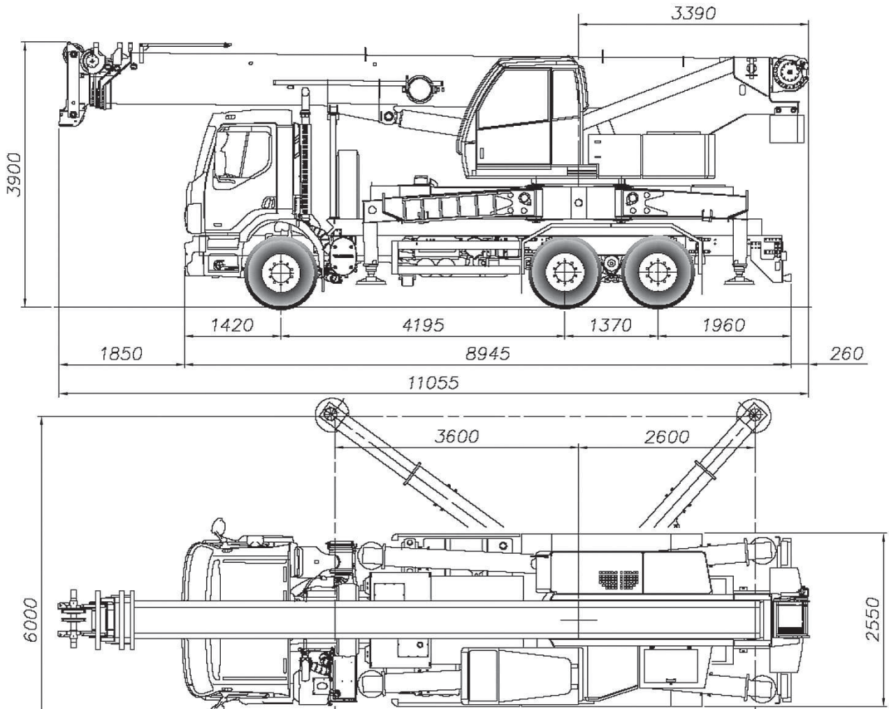
MTK 35 / VOLVO FEE 6x4 (Le dimensioni possono variare in funzione dell'autotelaio – Dimensions depending on chassis Les dimensions peuvent varier en fonction du châssis – Die Maße können je nach Fahrwerk variieren)
