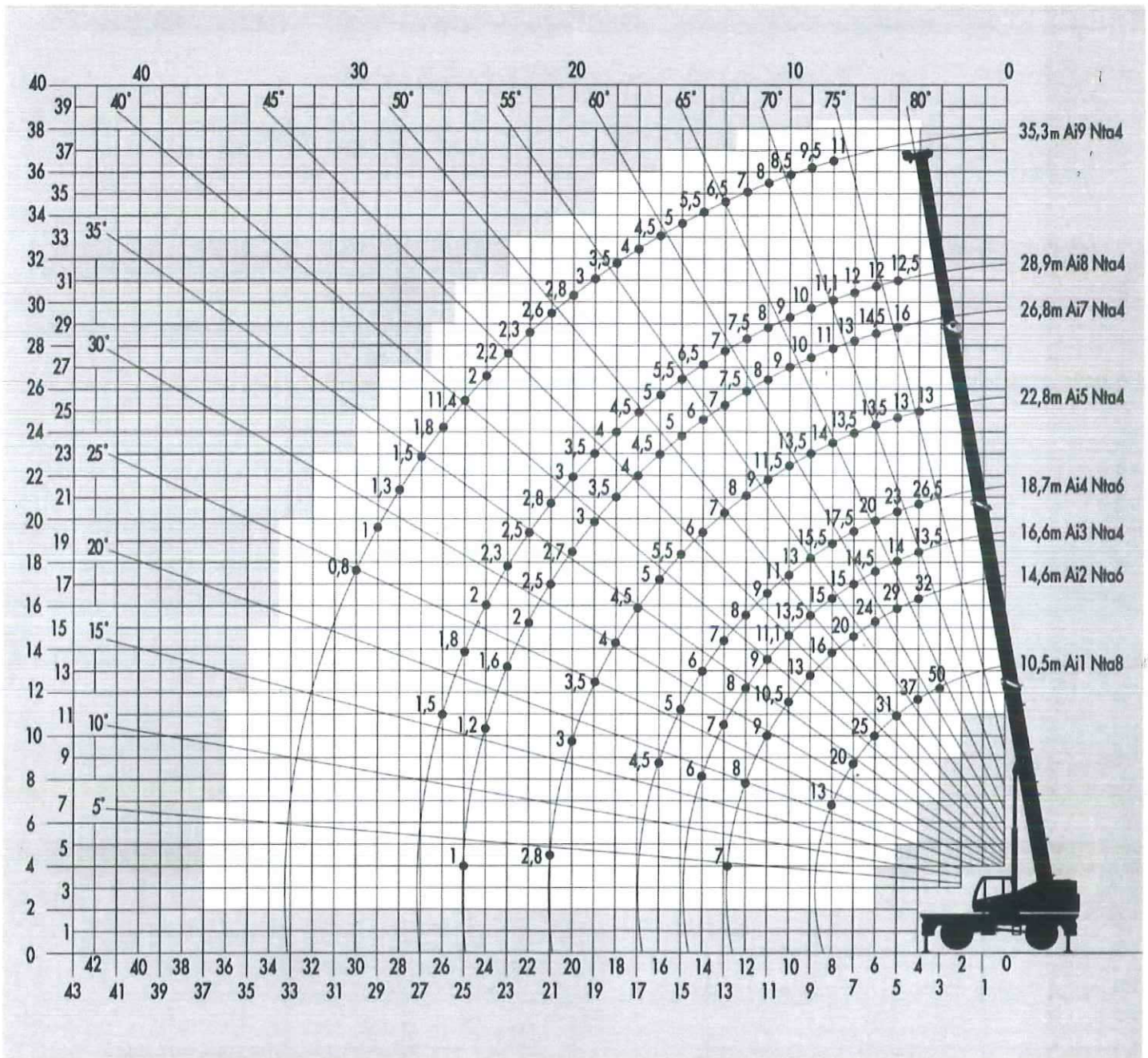
Diagramma portate su stabilizzatori su 360° - load chart on outriggers on 360°
